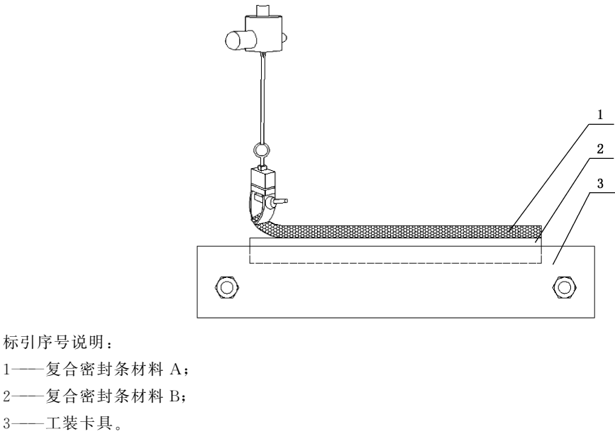
图 2 抗剥离性试验示意图
